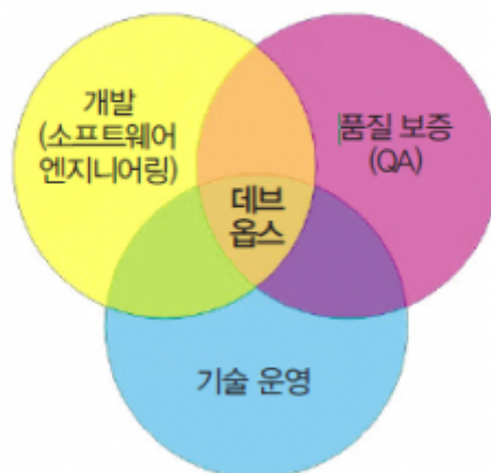
데브옵스의 개념
